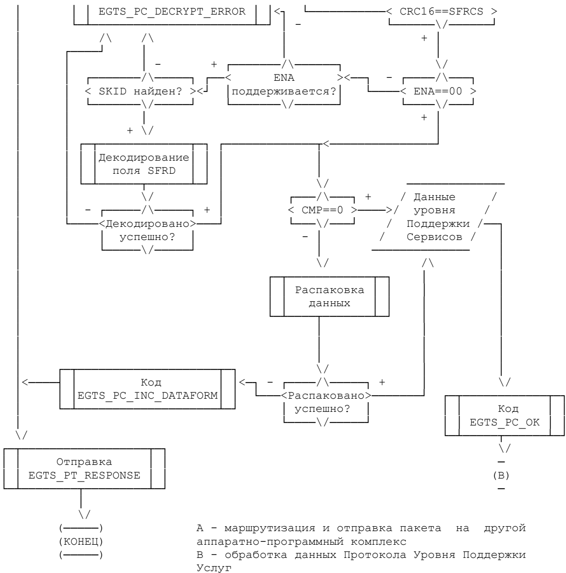
Рисунок 2. Блок-схема алгоритма обработки пакета данных протокола Транспортного уровня при приеме
